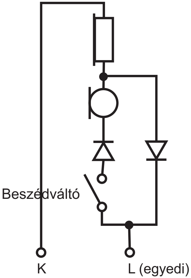
1+n diódás lakáskészülék
