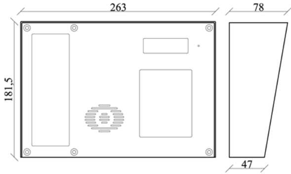
CODEfon™ -111 Esővédős falra szerelhető 1 névtáblás központ, kb 20 névhez
